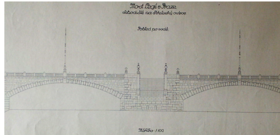
1924; Most Legii; Schodiště na Štřelecký ostrov - pohled po vodě
