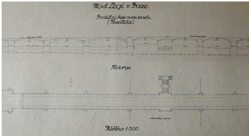
1924; Most Legii; Půdorys a podélný řez
