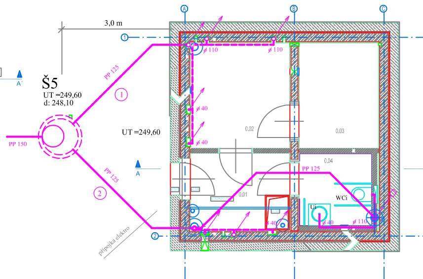
PŮDORYS 1.PP - KANALIZACE
